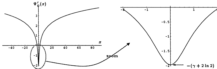
FIG. 2 – La fonction \Psi'_0(x) ( \gamma désigne la constante d'Euler \gamma \simeq 0,5772156649 \dots ).
