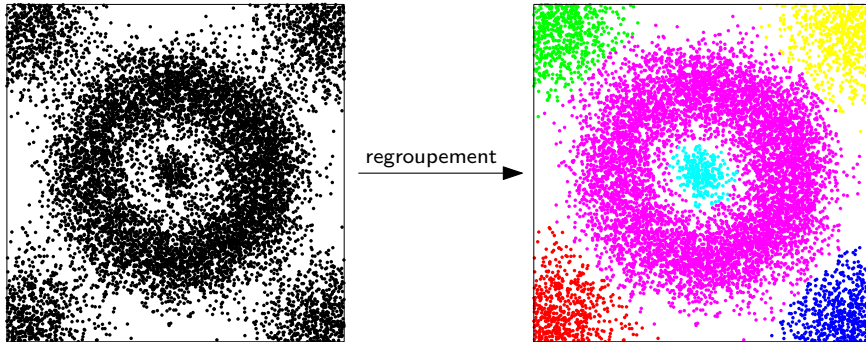
FIGURE 1. Un échantillon de points dans \mathbb{R}^2 (à gauche) et un regroupement de ces points (à droite).
