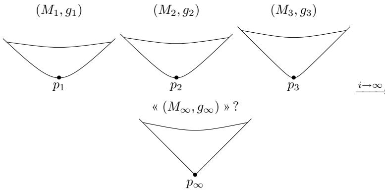
FIGURE 1.3. Sans borne sur la courbure, il n'y a pas convergence au sens de Cheeger-Gromov.
