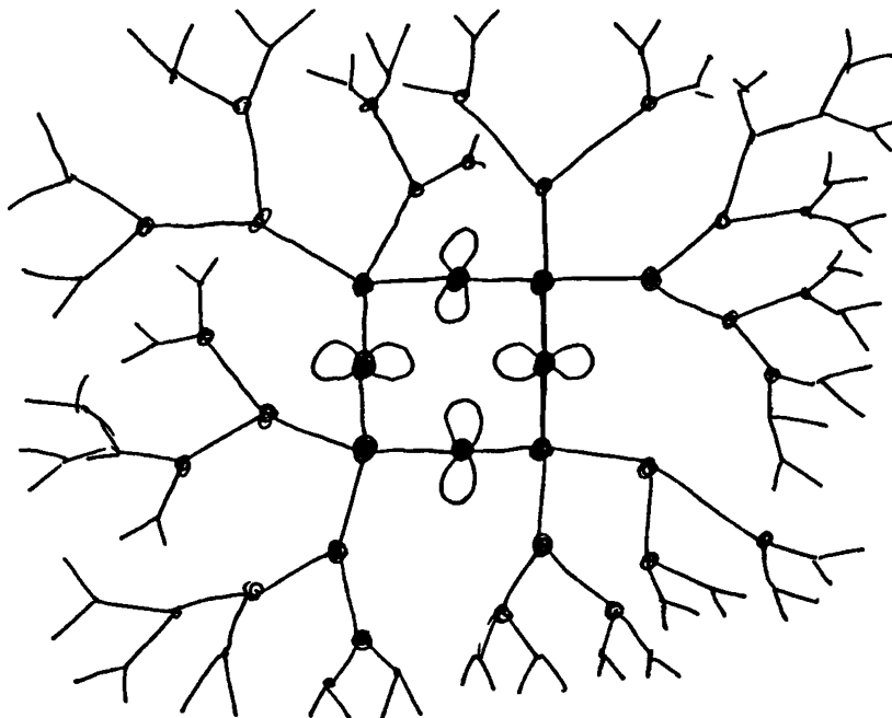
Le graphe T_1 .
